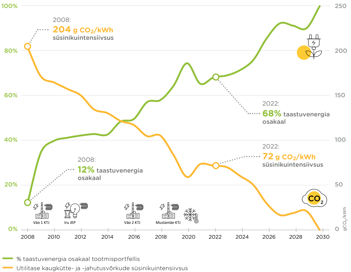
Joonis 13. Utilitase süsinikneutraalsuse kava eesmärgid [KTJ – koostootmisjaam; JEP – jäätmeeenergiaplakk]
