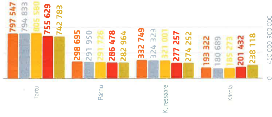
ELEKTRIENERGIA TARBIMINE kWh KURESSAARE, PÄRNU, KÄRDLA JA TARTU TARTU REGIONAALSES LENNUJAAMAS 2014–2018
