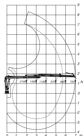
Bilden visar C 7,0 kran monterad på vår nya FARMA Generation 2 vagnsserie modell T 10.
