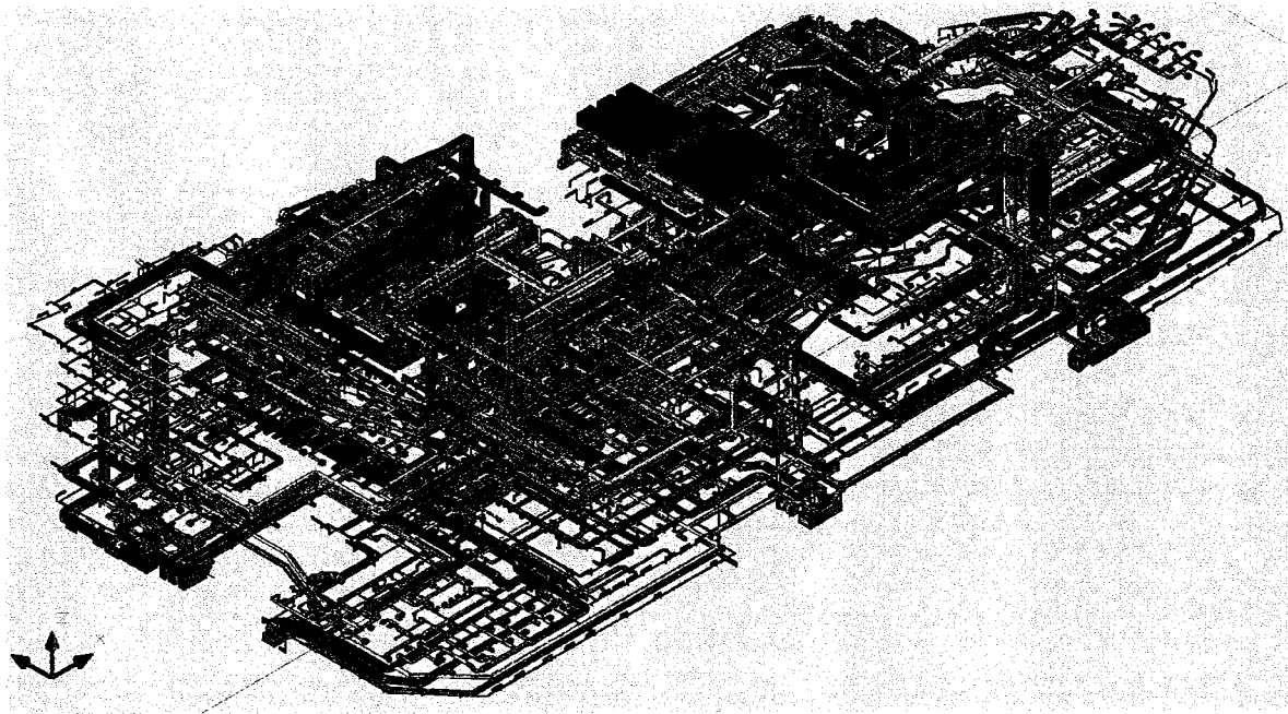
Pildil: Solaris keskus Tallinnas, kütte-ventilatsiooni-jahutuse koondmudel, teostatud programliga MagiCAD.
