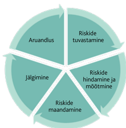
Joonis 3. Riskijuhtimisprotsess
